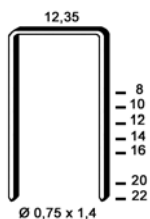
Série AK de 8 à 22 mm
